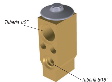
Válvula de expansión 2,0 TON
